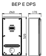
CAIXA PARA BARRA DE EQUIPOTENCIALIZAÇÃO PRINCIPAL (BEP) TIPO (POLIMÉRICO)
